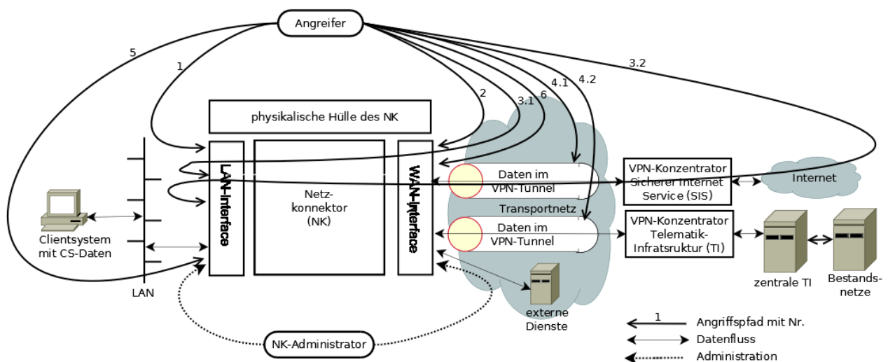
Abbildung 7: Externe Einheiten und Objekte im Zusammenhang, Angriffspfade
